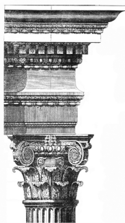
Детали римского композитного ордера
