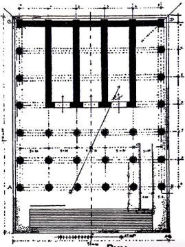
Рим Храм Юпитера Капитолийского К. 7-н. 6 в. до н.э.
