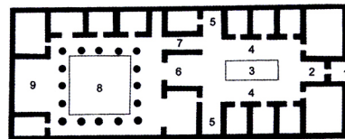
Римский жилой дом. Схема по Витрувию
