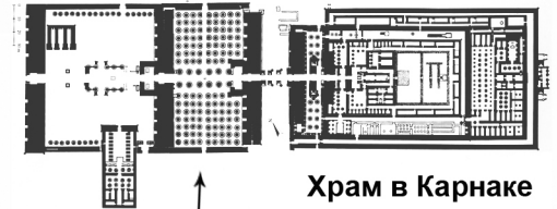
Гипостильный зал храма в Карнаке Новое царство
